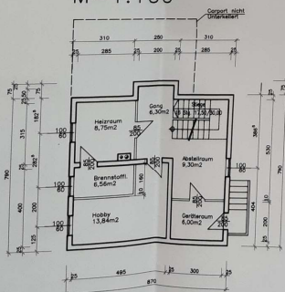
KELLERGEHOSS: M=1:100
