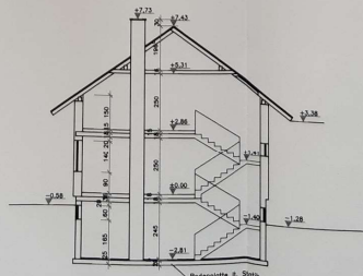
SCHNITT A-A M=1:100
